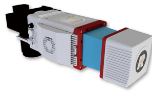
集成垂直下视的相机 例如: 索尼Alpha 6000 索尼 A7R III、索尼 A7R IV
